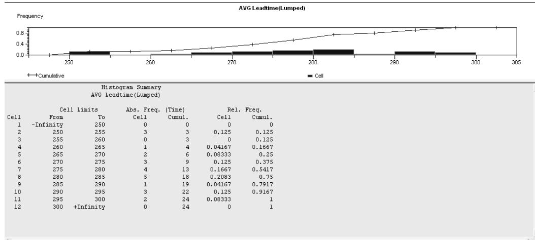
Figura 22 Histograma de Lead Time Actual
