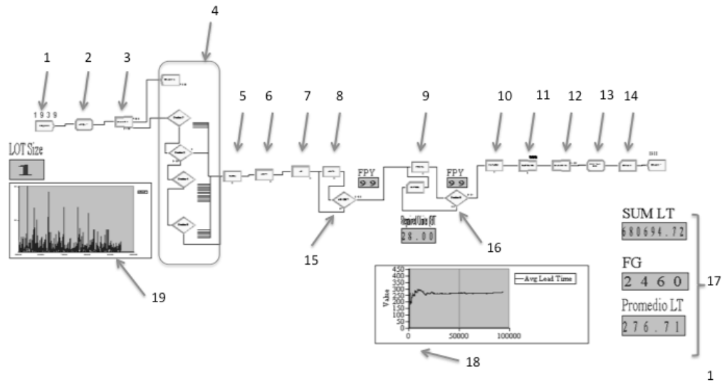
Figura 19 Modelo en Arena
