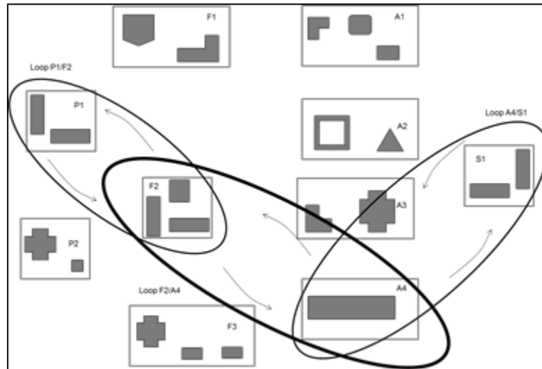
Figura 12 Flujo de Tarjetas POLCA
