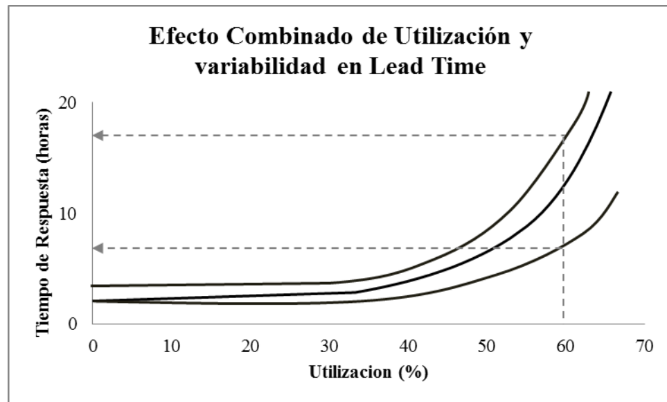
Figura 7 Efecto combinado de utilización y variabilidad sobre el lead time.
