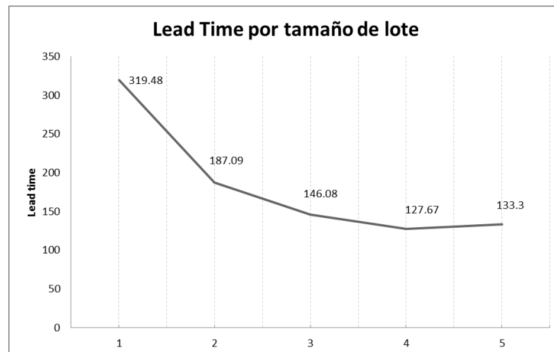
Figura 25 Lead time por tamaño de lote (Arena)
