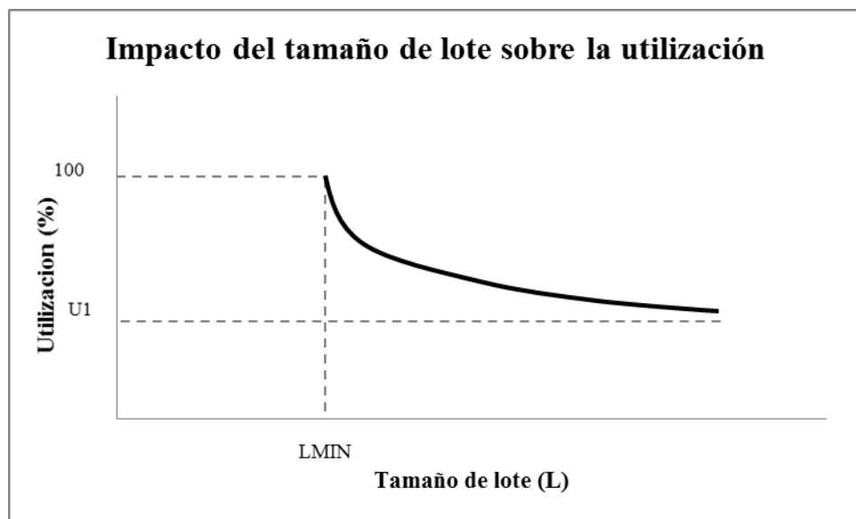
Figura 8 Impacto del tamaño de lote sobre la utilización
