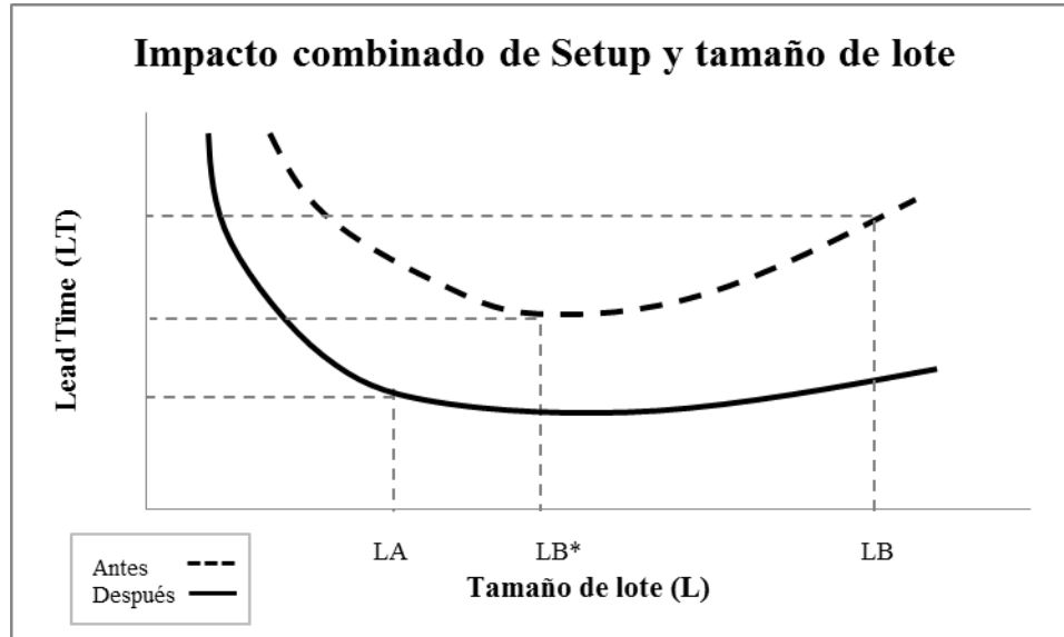
Figura 10 Impacto combinado de setup y tamaño de lote
