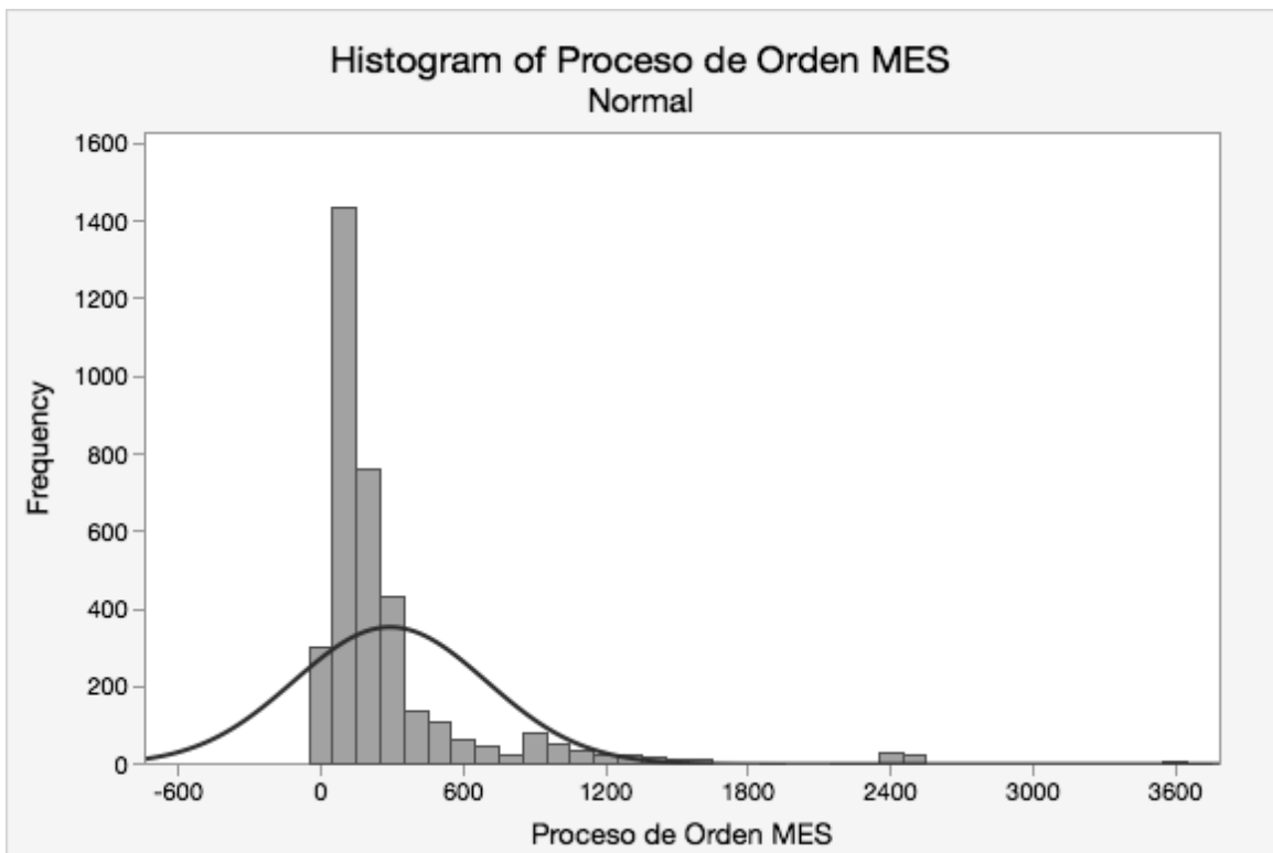
Figura 18 Histograma de frecuencias Lead time actual
