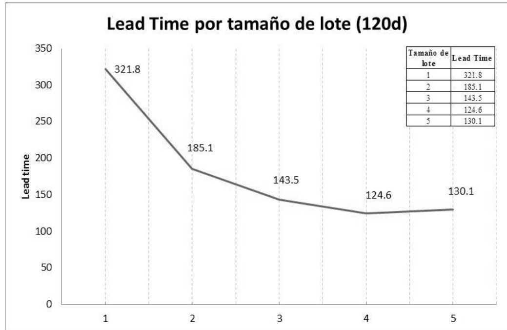
Figura 27 Lead time por tamaño de lote (Arena) 120 días.
