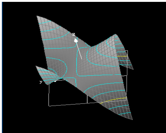
Figura 2. Líneas de contorno para la función z = \cos(x) - y + 3x^2 \text{sen}(y)
