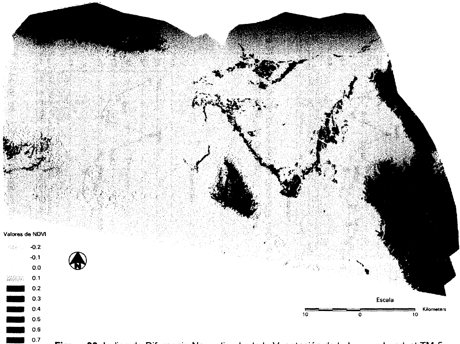
Figura 30. Índice de Diferencia Normalizada de la Vegetación de la Imagen Landsat TM-5 de Octubre de 1995
