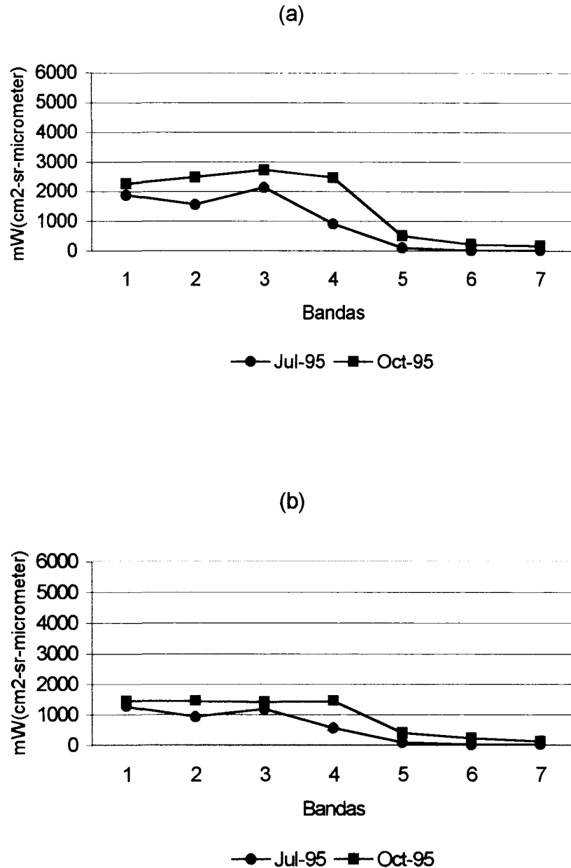
Figura 20. Valores de radianza del Matorral Desértico Micrófilo. Cuadrantes de muestreo 1 y 7 (a y b respectivamente).
