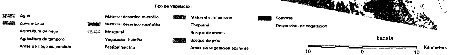
Figura 16. Clasificación de la Imagen Landsat TM-5 de Octubre de 1995
