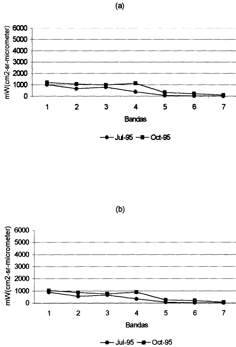
Figura 28. Valores de radianza del matorral submontano, Cuadrantes de muestreo 15 y 16 (a y b respectivamente).
