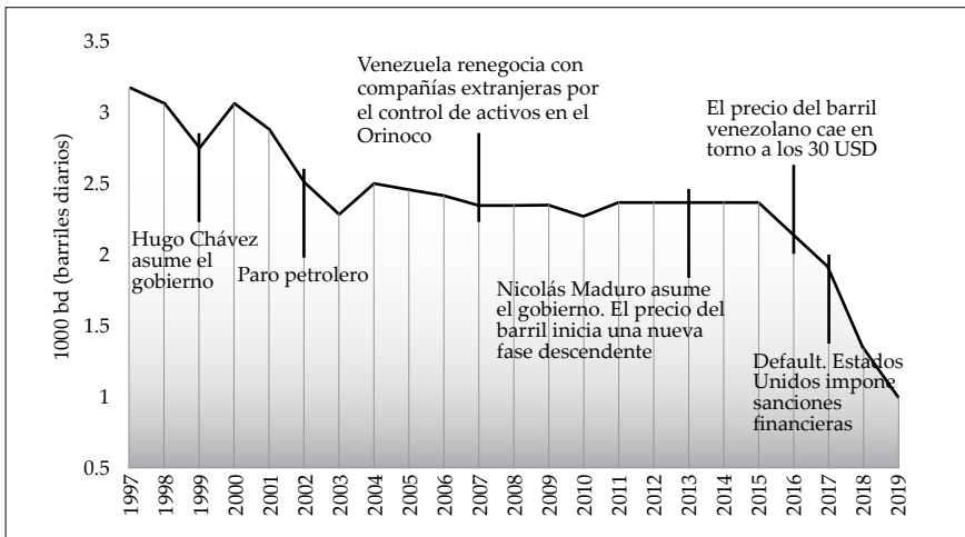
GRÁFICA 5. VENEZUELA. PRODUCCIÓN DE PETRÓLEO (1997-2019)
