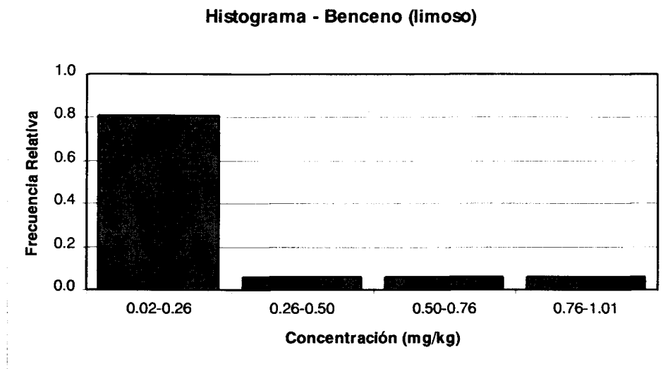
Fig. 4.4 Distribución de concentraciones de benceno en suelo limoso
